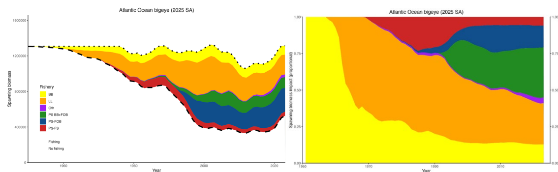
Figure 19.30.1. Diagramme d'impact estimé sur la biomasse du stock reproducteur escomptée (t) de thon obèse par chacune des principales pêcheries des flottilles/engins sur la base du modèle de référence de l'évaluation de SS de 2025 (panneau de gauche). La ligne hachée supérieure indique la SSB escomptée dans le cadre de l'absence de pêche, tandis que la ligne hachée inférieure indique la tendance de la SSB avec toute la
