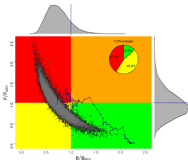
Figure 1. Diagramme de Kobe pour les trajectoires de l'état du stock d'espadon de la Méditerranée pour les distributions a posteriori combinées en 2018, estimées lors de l'évaluation du stock en 2020. Le diagramme circulaire inséré indique la probabilité que le stock se situe dans chaque quadrant de couleur de Kobe. Les distributions de probabilité indiquées sur chaque axe représentent l'incertitude entourant B/B_{PME} et F/F_{PME} actuelles. La ligne noire indique la trajectoire de l'état du stock à partir de 1950.
