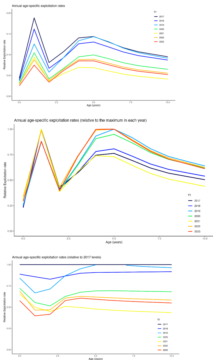
Figure 19.30.3. Schémas des récentes estimations des taux d'exploitation par âge du thon obèse de l'Atlantique sur la base du cas de référence du modèle. Panneau supérieur : estimations « brutes » ; panneau du milieu : estimations mises à l'échelle pour chaque année en fonction de l'âge auquel le taux d'exploitation est le plus élevé ; et panneau inférieur : estimations mises à l'échelle pour chaque âge en fonction de la valeur de l'âge en question pour 2017.
